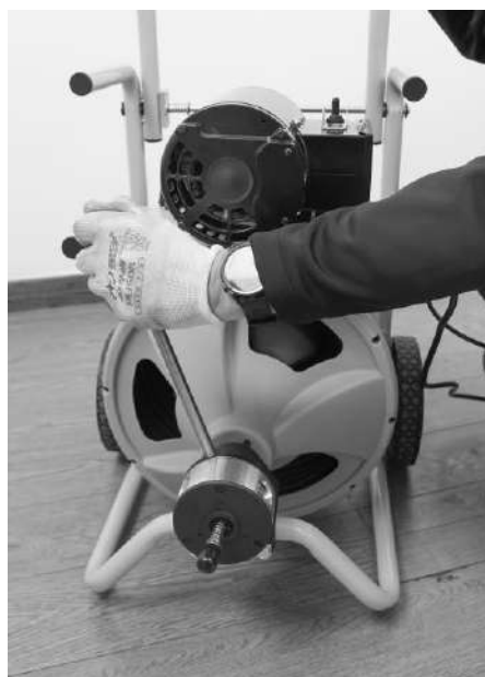
Рис 6 – В рабочем положении, подаваемая вручную спираль
